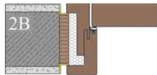
Zargensystem (2B) INTRA-UZ-ALU 40-52 TS40 Wandbündiges Zargensystem 2-schalige Zarge mit Unterzarge und Alu-Anputzprofil Spiegelbreite 40mm / 52mm
