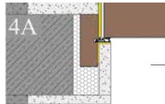
Zargensystem (4A) FLAT VD verdecktes, völlig in die Wand integriertes Zargensystem Verdeckter Blockrahmen mit Alu-Schutzprofil
