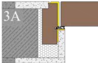
Zargensystem (3A) FLAT ALU-20 TS48 Wandbündiges Zargensystem Verdeckter Blockrahmen mit Alu-Schutzprofil. Spiegelbreite 20mm
