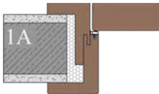
Zargensystem (1A) INTRA 63-75 TS40 Wandüberstehendes Zargensystem 2-schalige Zarge auf der Wand Spiegelbreite 63mm / 75mm
